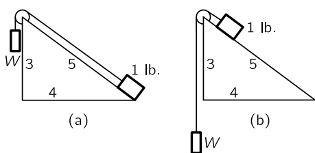
图 4.3: 斜面
