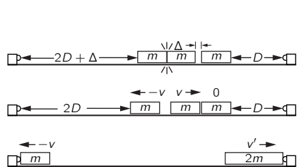
图 10.6: 验证以速度 v 运动的质量为 m 的物体与一个质量相同的静止物体碰撞后结合在一起以质量 2m 、速度 \frac{v}{2} 运动的实验
