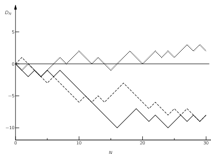
图 6.5: 无规行走取得的进度。横座标 N 表示所走的步子总数；纵座标 D_N 表示离开起点的净距离
