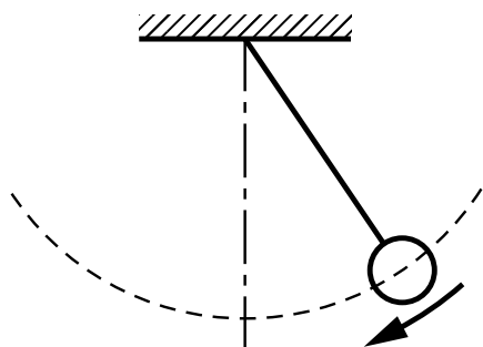
图 4.7: 单摆
