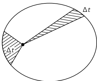
图 7.2: 开普勒的面积定律
