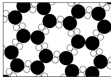
图 1.4: 冰
