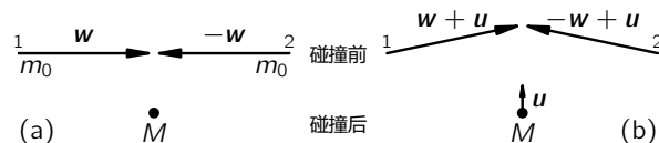
图 16.4: 质量相同的物体之间的非弹性碰撞的两种看法
